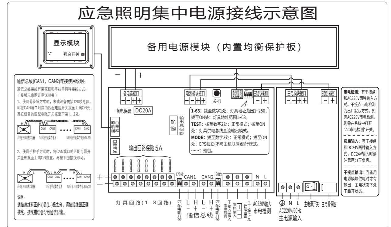
150/200W 应急照明集中电源接线示意图
