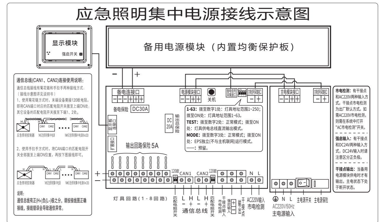
300W 应急照明集中电源接线示意图
