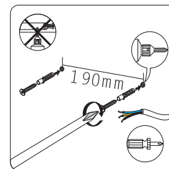
根据后板孔位在墙体钻孔，并安装好堵塞和沉头螺丝
